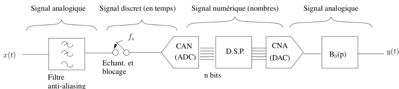
Figure 1 : Schéma d'une chaîne d'acquisition numérique de l'information
