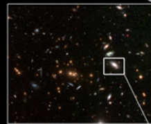
Amas de galaxies
